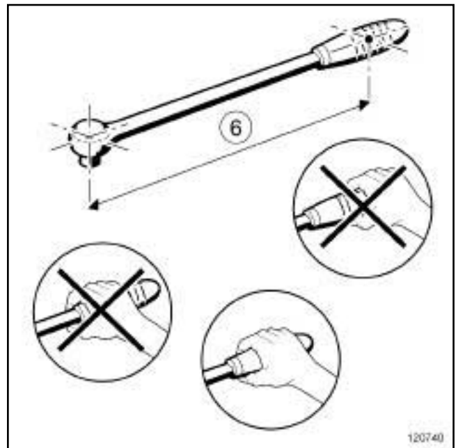
(6) плечо рычага
